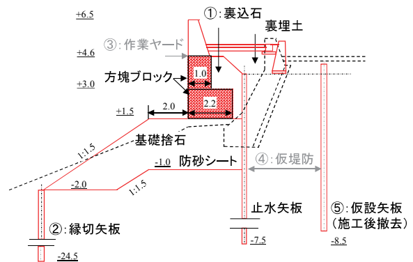
図-2 設定した護岸改良断面例(方塊式ブロック工法)
