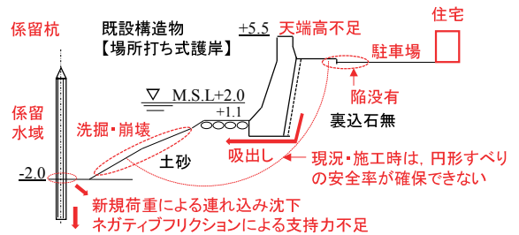
図-1 改良対象とした既設護岸断面図
