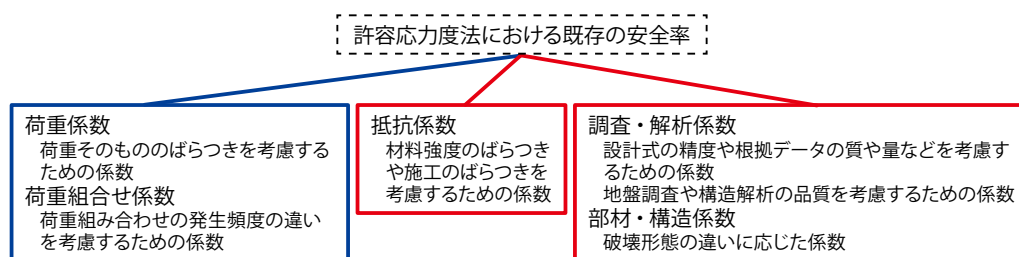
図 許容応力度法と部分係数設計法
